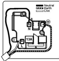
Wiring
