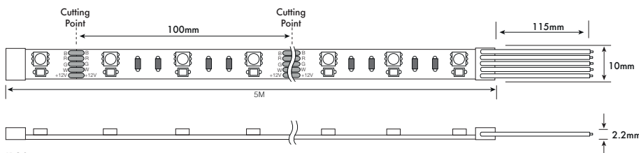
IP20
