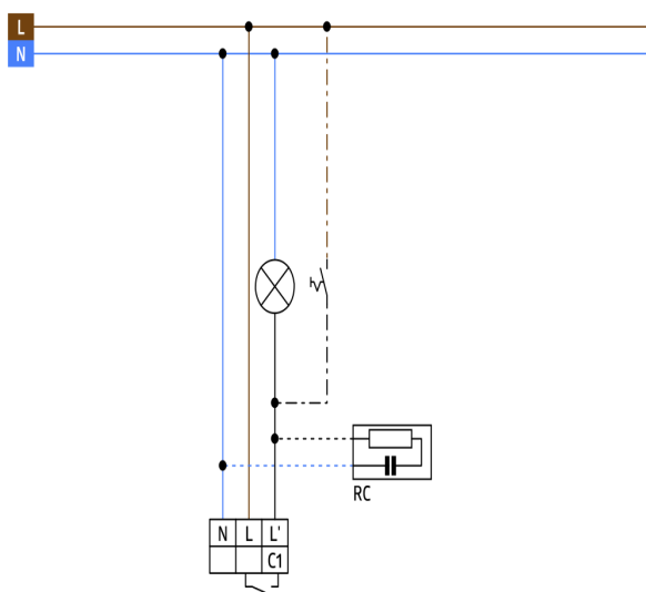
Wiring diagrams
