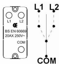
Wiring
