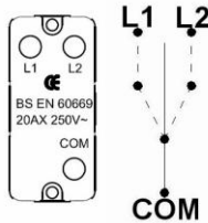
Wiring
