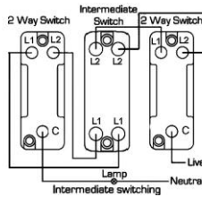
Wiring
