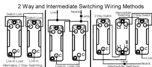
Wiring
