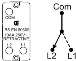
Wiring
