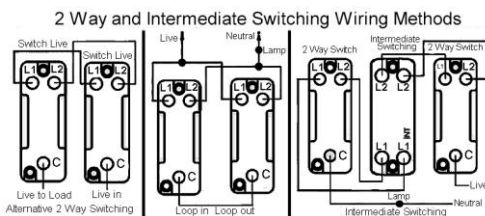
Wiring
