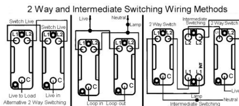
Wiring
