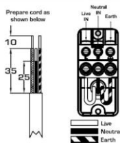
Wiring
